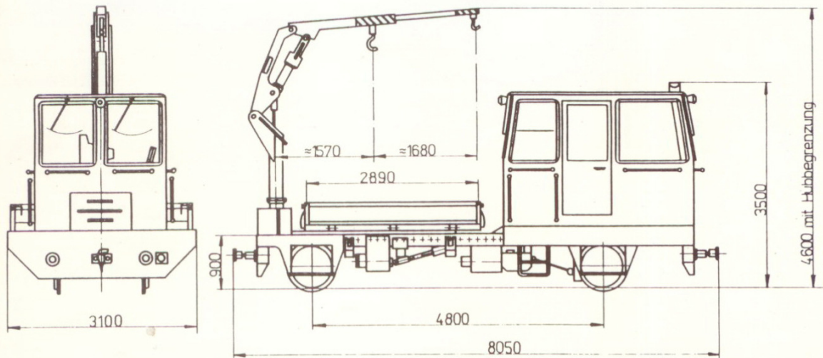
Übersichtszeichnung - MZG -
